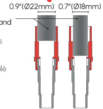
Rigid pipe Starres Rohr | Tube rigide
