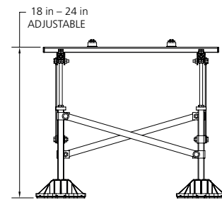
Mini Frame – Tall BN8100/1 & Extension Kit – Tall BN8101/1
