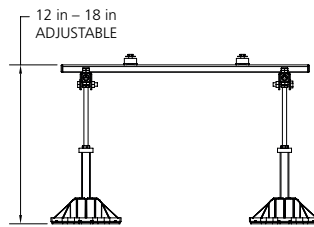
Mini Frame BN8100 & Extension Kit BN8101
