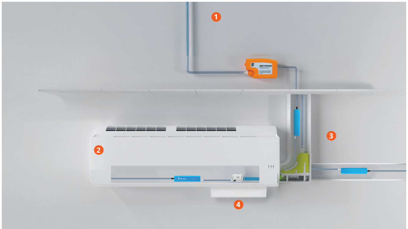
1 An der Decke 2 In der Klimaanlage 3 Innerhalb des Kanalsystems 4 Unter der Einheit
