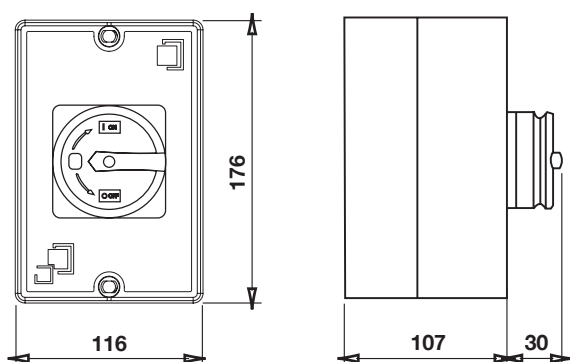
Grand modèle 4 pôles, 40-63 A
