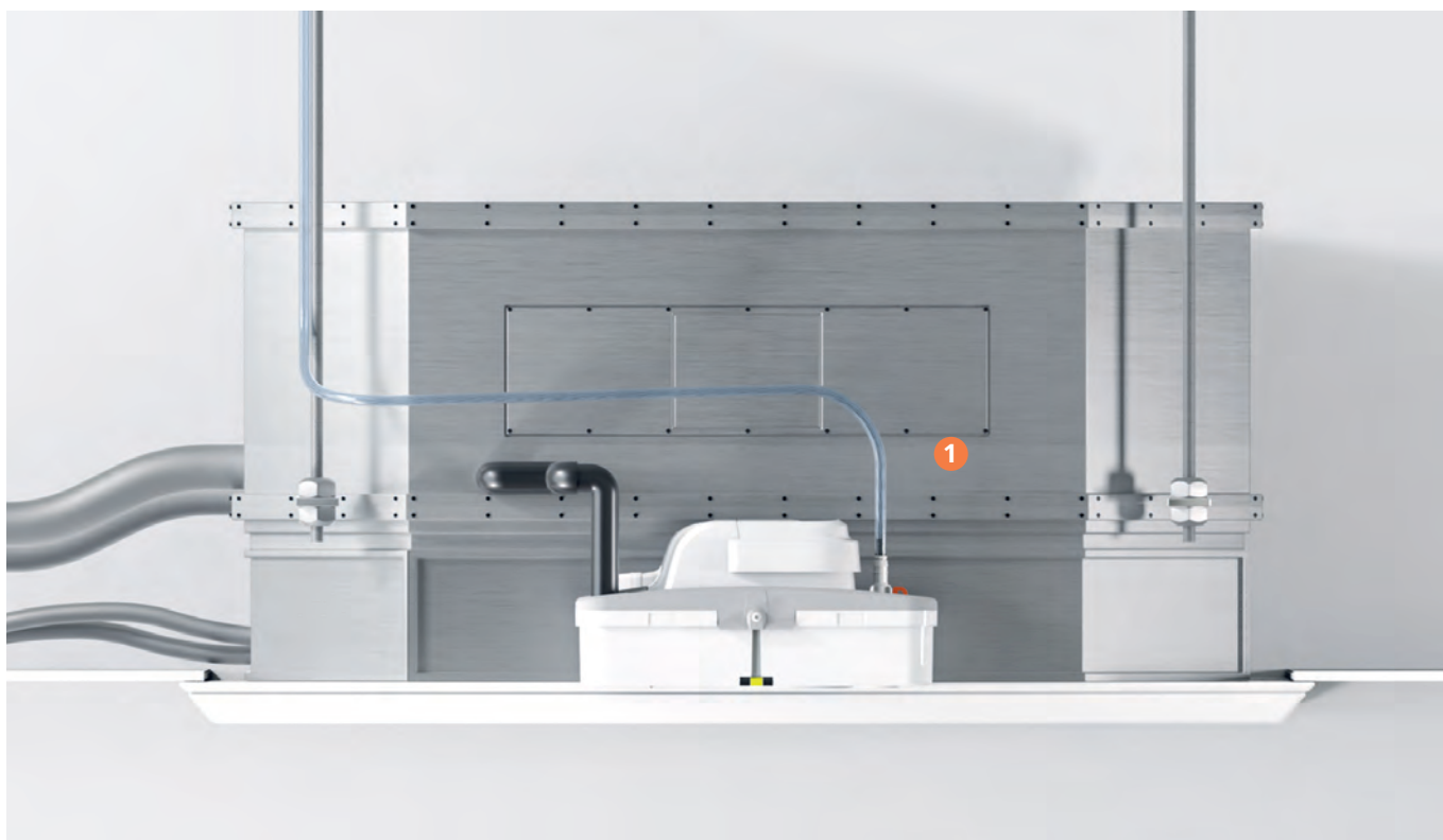
1 Pompe Max Hi-Flow vissée sur une cassette.
