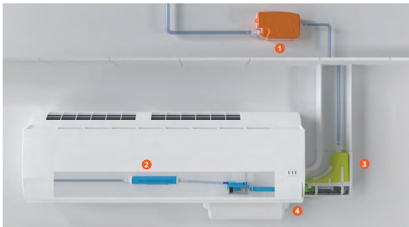
1 Au plafond (Remarque: support antivibratoire) 2 Dans le climatiseur 3 À l'intérieur de la goutlotte 4 Sous l'unité
