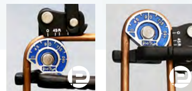
Conception à double charnière
