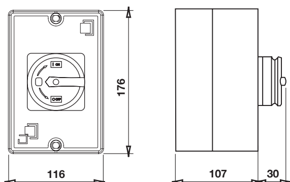
Grand modèle 4 pôles, 40-63 A
