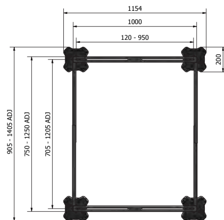
BN8411 Maxi Châssis Poids: 16 kg
