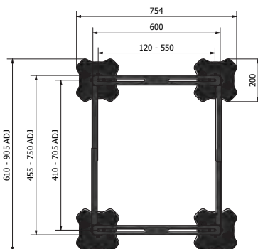
BN8410 Micro Châssis Poids: 11.5 kg
